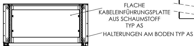
ABSCHNITT I-I
