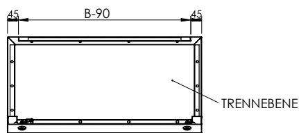
ABSCHNITT H-H
