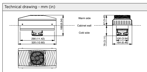
KTCU502440IP55 KLIMAGERÄT TE 50W IP55
