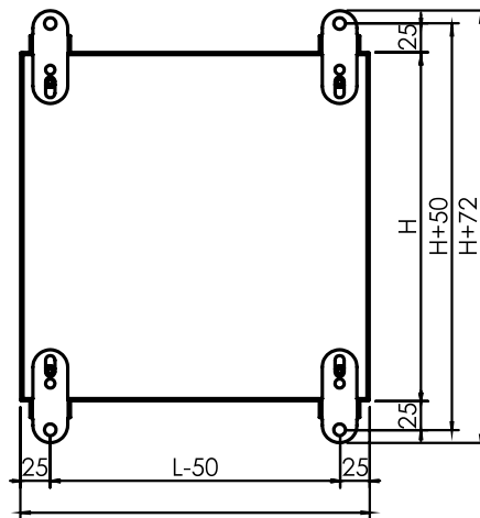
Montage der FLACHEN Wandbefestigungshalter an das Wandgehäuse
