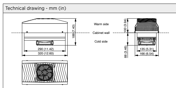
KTCU1002440IP55 KLIMAGERÄT TE 100W IP55
