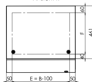
ANSICHT K
