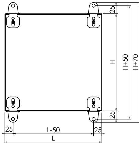
Montage der ERHÖHTEN Wandbefestigungshalter an das Wandgehäuse
