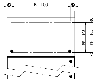
ANSICHT K 22°
